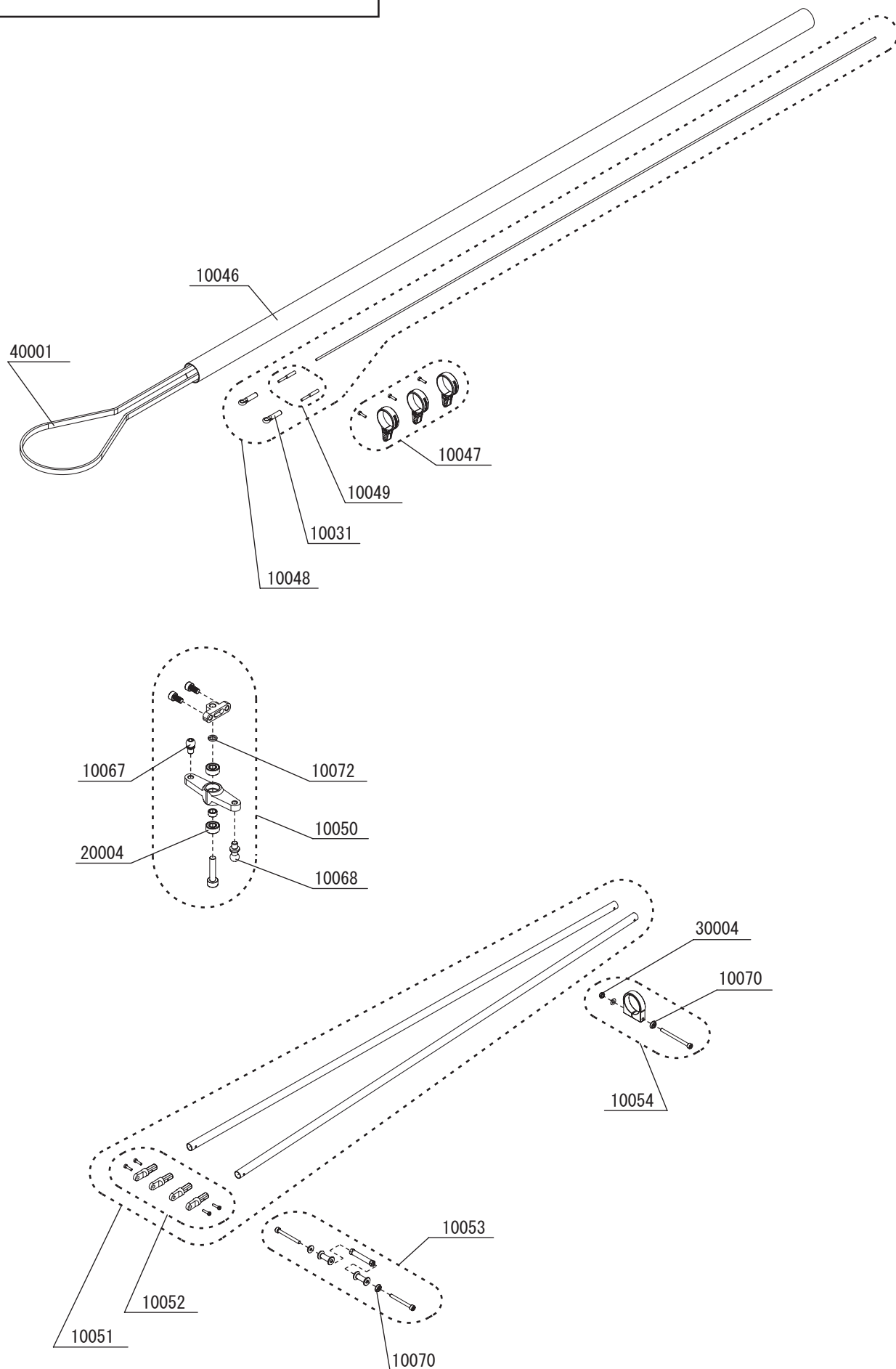
パーツ図 5 テール
